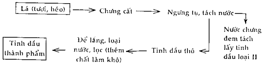
Hình 3.2. Quy trình sản xuất tinh dầu sả
