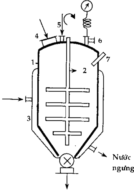
Hình 8.5. Nồi thơm hóa và đường hóa 1-thân nồi; 2-cánh khuấy (= 30-40v/phút); 3-vỏ hơi; 4-cửa cho nguyên liệu; 5-ống nước; 6-van 3 ngã dùng cầm áp kế và xả khí; 7-ống cắm nhiệt kế
