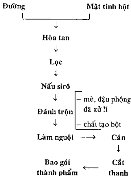
Hình 9.4. Sơ đồ sản xuất kẹo thanh
