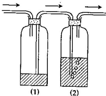
Hình 14.4. Bộ bình hứng nước và ngăn lửa
