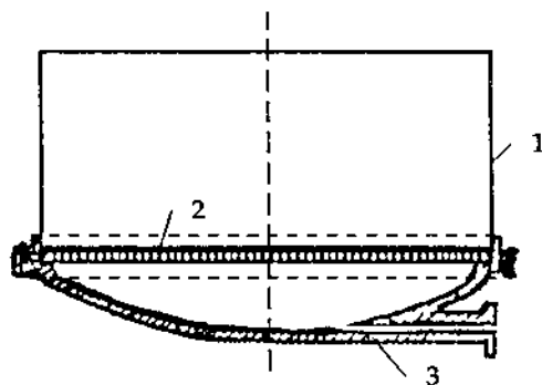
Hình 4.4 Máy lọc thùng hút 1-bên chứa; 2-màng lọc; 3-ống xả
