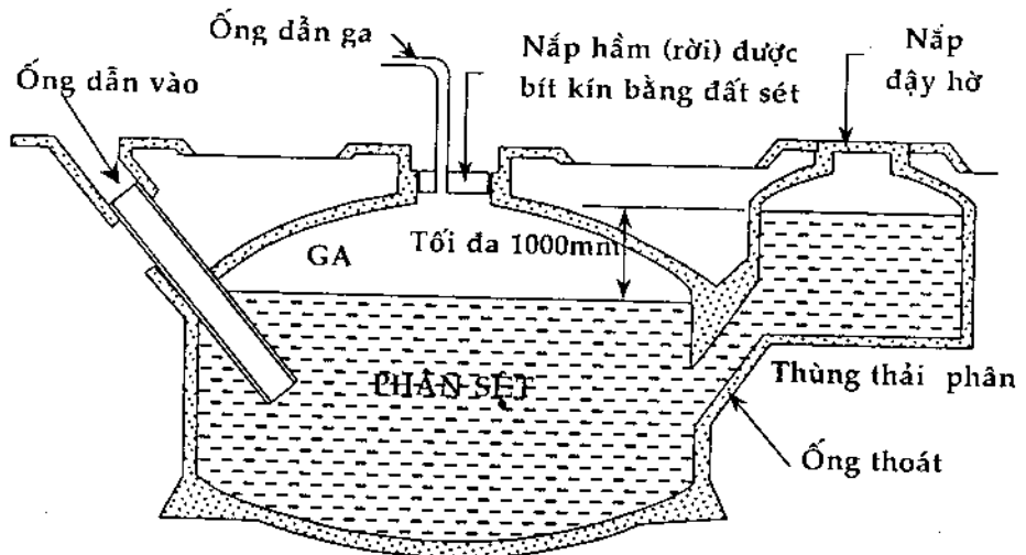
Hình 14.2. Loại hầm ủ vòm cố định hình tròn
