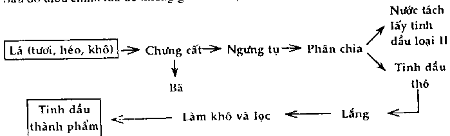
Hình 3.3. Công nghệ sản xuất tinh dầu bạc hà.
