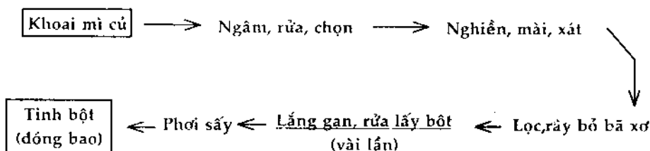
Hình 2.3. Sơ đồ sản xuất tinh bột khoai mì.
