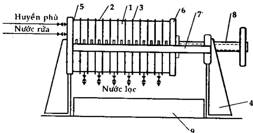
Hình 2.6. Máy lọc khung bản
