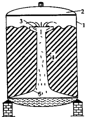
Hình 11.1. Nồi nấu thủ công 1-Thân nồi, dày 4-6mm; 2-Nắp; 3-Hoa sen; 4-Ống tuần hoàn Ø80-100mm; 5-Đáy giã có nhiều lỗ Ø6-12mm
