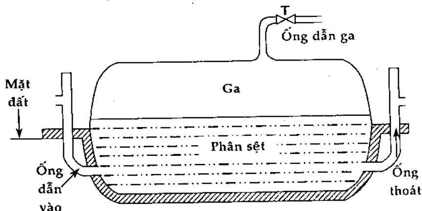
Hình 14.3. Hầm ủ bằng túi dẻo
