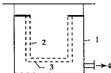
Hình 8.1. Thùng lọc sirô 1- thân thùng lọc; 2- lưới lọc thô có đường kính lỗ d=3-5\text{mm} ; 3- lưới lọc tinh có đường kính lỗ d=1-2\text{mm} ; 4- van tháo sirô và nước vệ sinh
