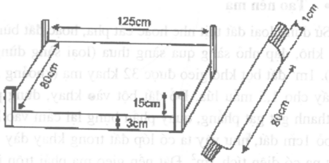
Hình 39. khay mạ và thanh gạt
